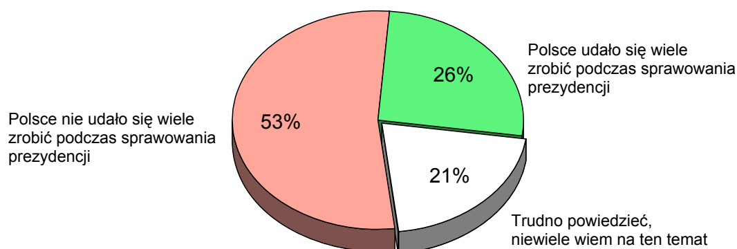
RYS. 2. W GRUDNIU ZAKOŃCZYŁO SIĘ PÓLROCZNE PRZEWODNICTWO (PREZYDENCJA) POLSKI W RADZIE UNII EUROPEJSKIEJ. JAK PAN(I) OCENIA POLSKĄ PREZYDENCJĘ? CZY, PANA(I) ZDANIEM:
